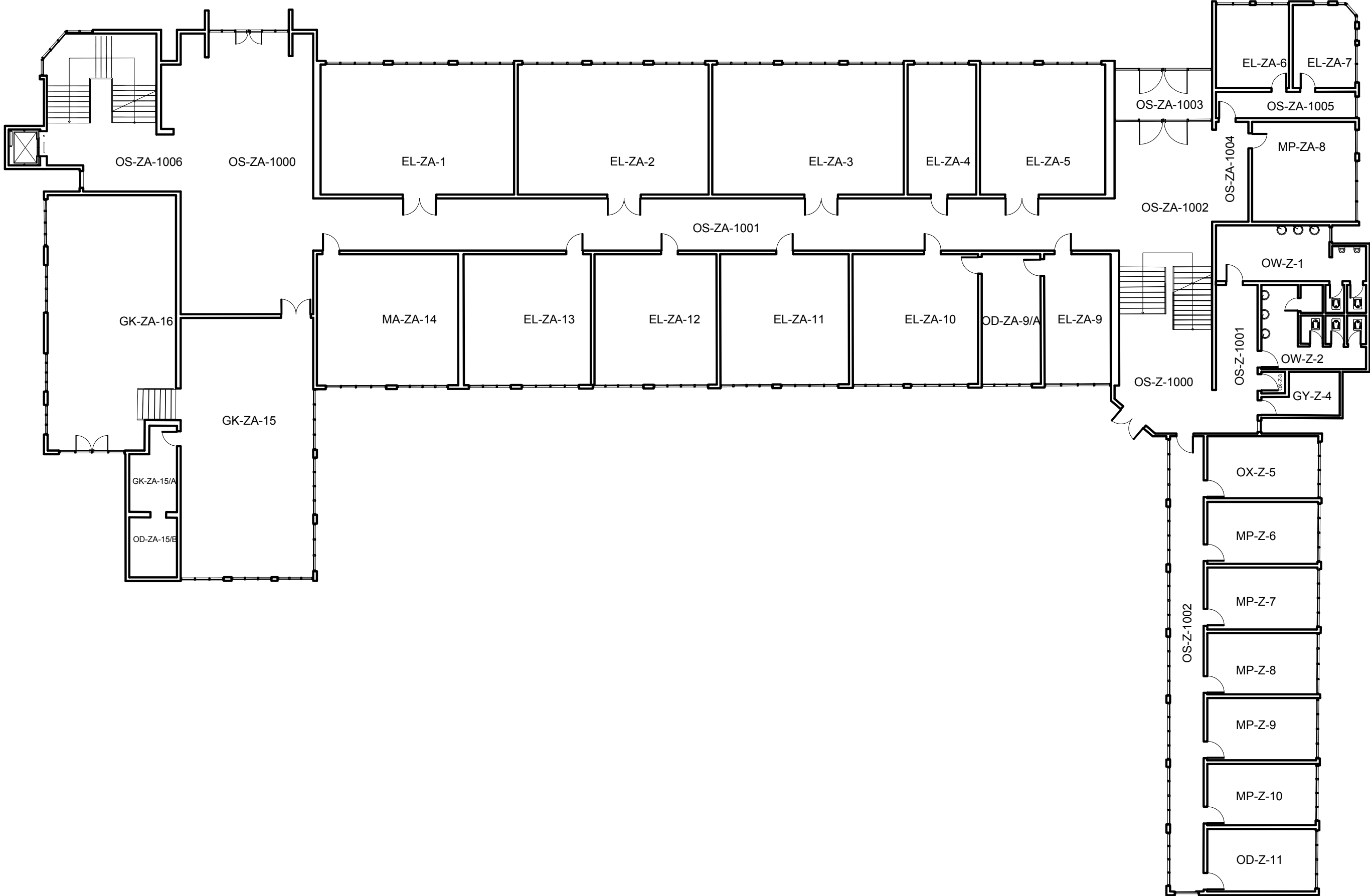
ZEMİN KAT PLANI
